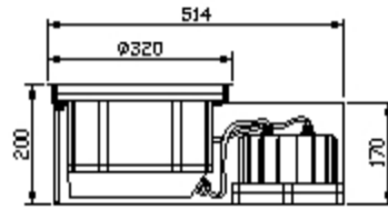
C: 70W-150W分体式尺寸图
