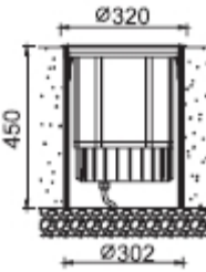
B: 250W 一体式尺寸图
